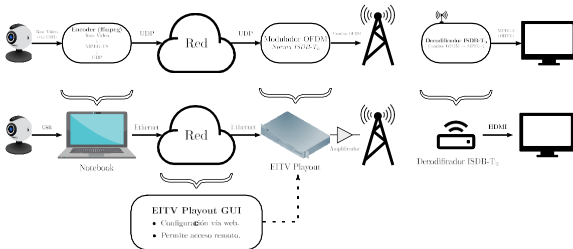
Figura 1: Diagrama lógico (arriba) y físico (abajo) de la transmisión.
