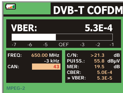
Figure 30.- Écran de mesure du BER de signaux modulés en COFDM. VBER.
