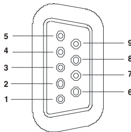
Figura 42.- Conector RS-232C. Vista exterior.
