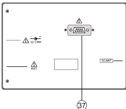
Figure 8.- Panneau postérieur.
